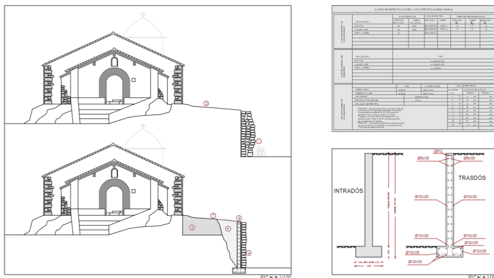
Figura 1. Plano técnico del proyecto: actuación prevista para el nuevo muro de contención.
